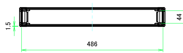
A-A ( 1:6.5 )
