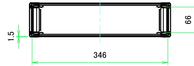
A-A (1:6)
