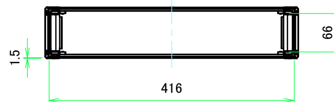
A-A (1:6.5)
