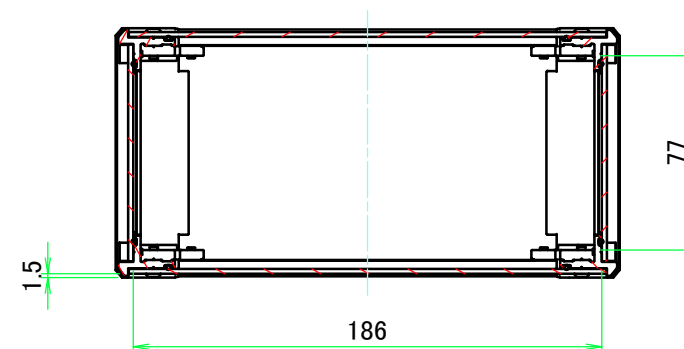
A-A (1:3)
