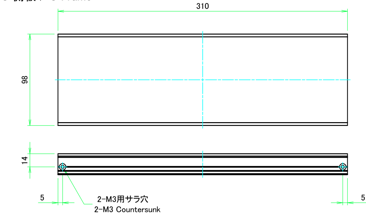
※ 反対面も同様 / Same on the other side. 表面 / Front side
