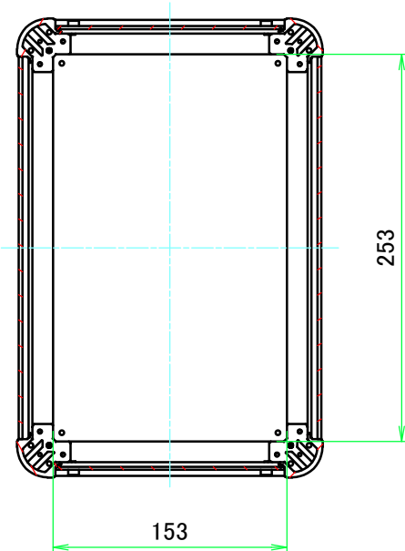
B-B ( 1 : 4.5 )
