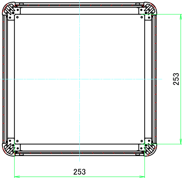
B-B ( 1 : 4.5 )
