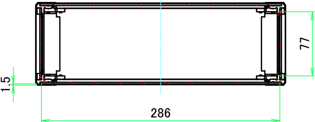
A-A ( 1 : 4.5 )
