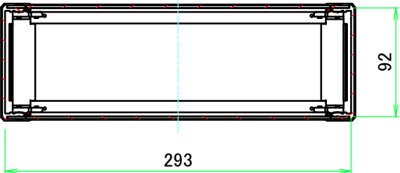
C-C ( 1 : 4.5 )
