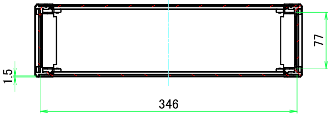
A-A (1:5)
