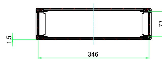
A-A ( 1 : 6 )
