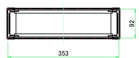
C-C ( 1 : 6 )
