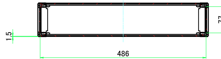
A-A ( 1 : 6.5 )
