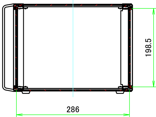
A-A (1:6)
