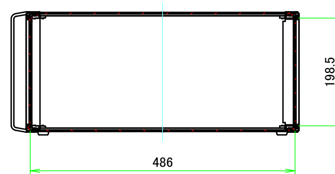
A-A (1:7)
