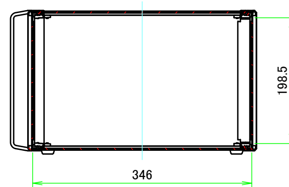
A-A (1:6)
