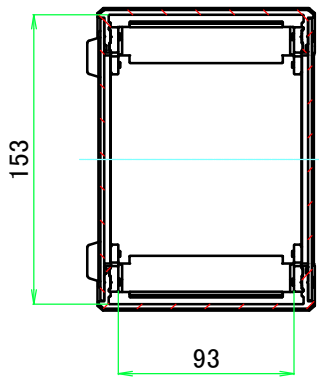
A-A ( 1 : 4 )
