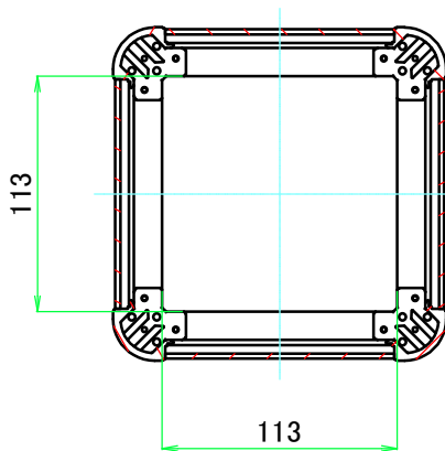
C-C ( 1 : 4 )
