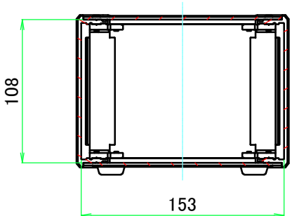
B-B ( 1 : 4 )
