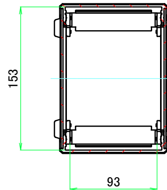
A-A ( 1 : 4 )
