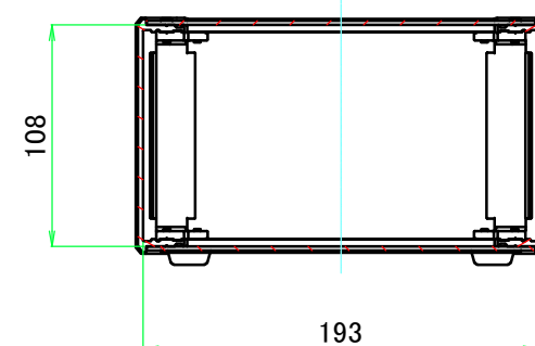
B-B ( 1 : 4 )
