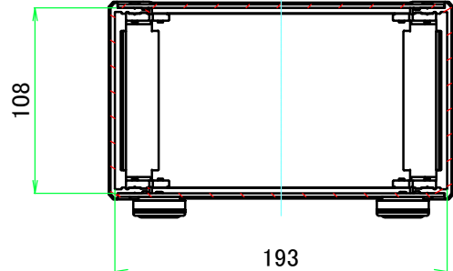
A-A ( 1 : 4 )
