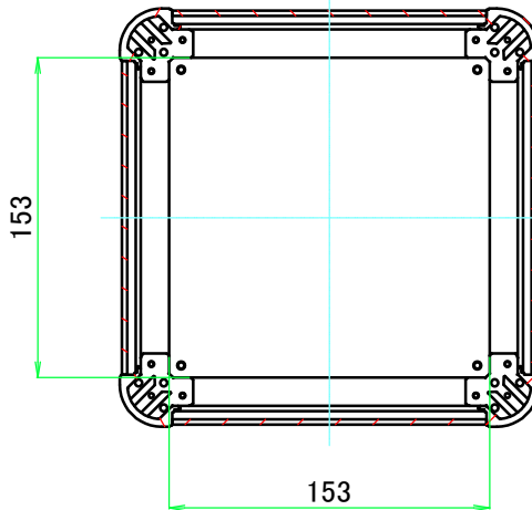
C-C ( 1 : 4 )
