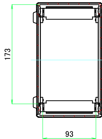
A-A (1:4)
