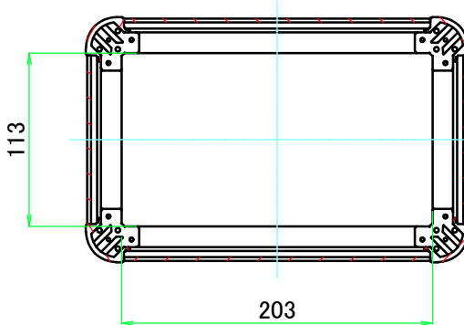
C-C ( 1 : 4.5 )
