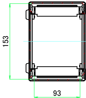
A-A ( 1 : 4.5 )
