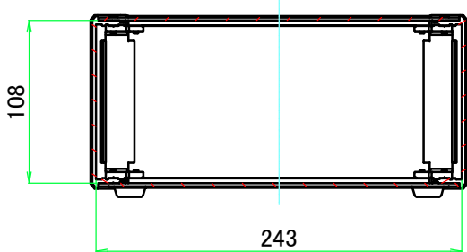
B-B ( 1 : 4.5 )
