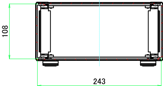
A-A ( 1 : 4.5 )
