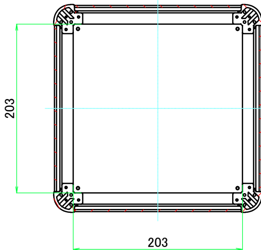
C-C ( 1 : 4.5 )
