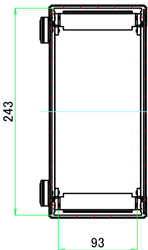
B-B ( 1 : 4.5 )
