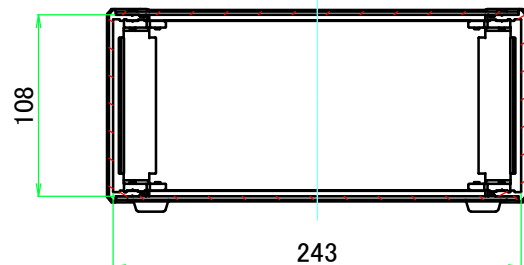
B-B ( 1 : 4.5 )
