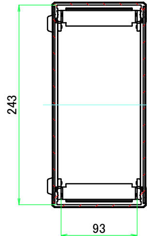
A-A ( 1 : 4.5 )
