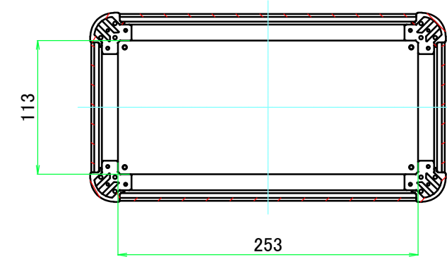
C-C ( 1 : 4.5 )
