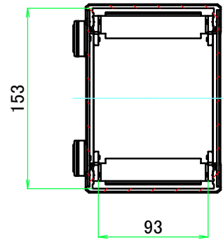
B-B ( 1 : 4.5 )
