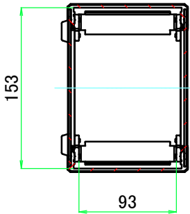
A-A ( 1 : 5 )
