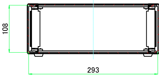
B-B ( 1 : 5 )
