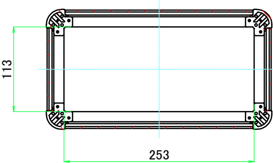
C-C ( 1 : 5 )
