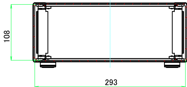
A-A ( 1 : 4.5 )
