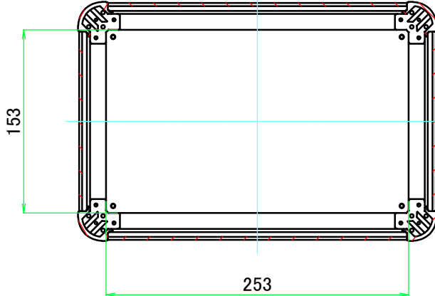
C-C ( 1 : 4.5 )
