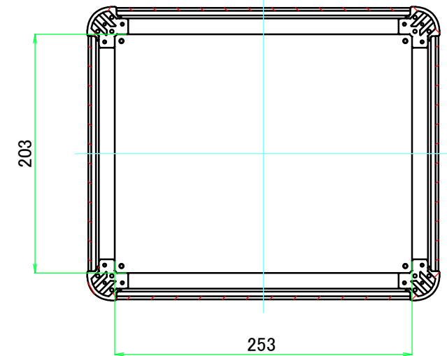
C-C ( 1 : 4.5 )
