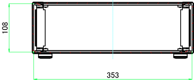
A-A ( 1 : 5 )
