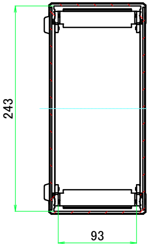
A-A ( 1 : 4.5 )
