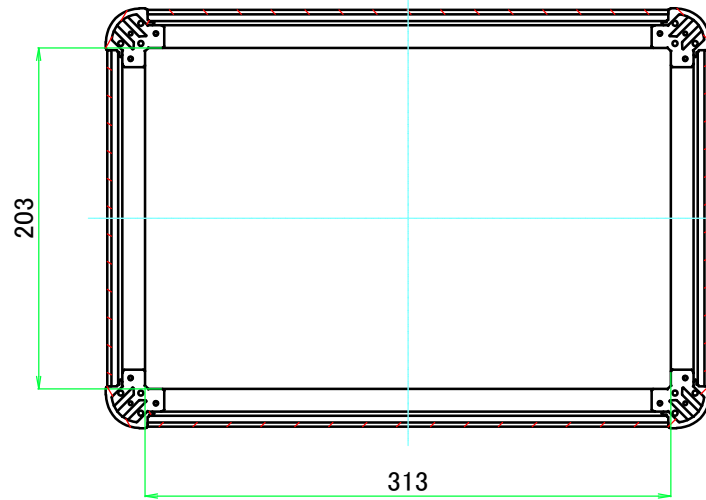
C-C ( 1 : 4.5 )
