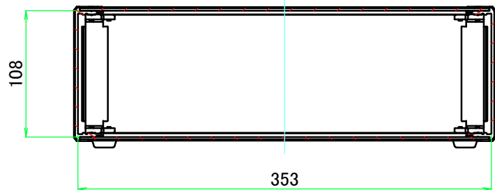
B-B ( 1 : 4.5 )
