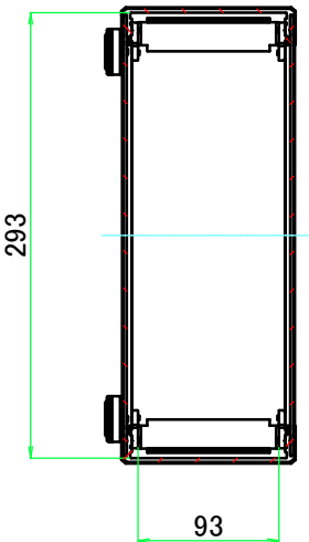
B-B ( 1 : 5.5 )
