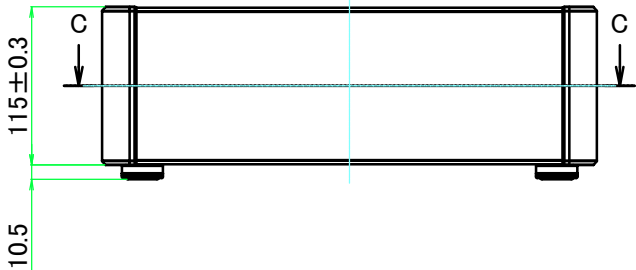
A-A ( 1 : 5.5 )
