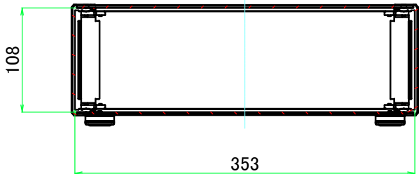
A-A ( 1 : 5.5 )
