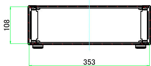
A-A ( 1 : 6.5 )
