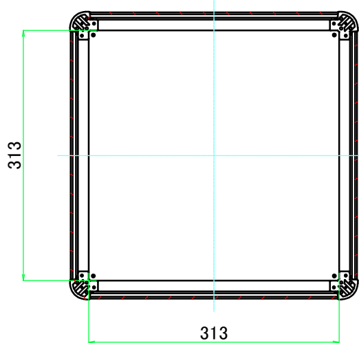
C-C ( 1 : 6.5 )
