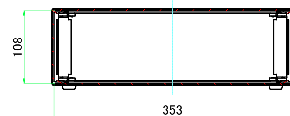
B-B ( 1 : 5.5 )
