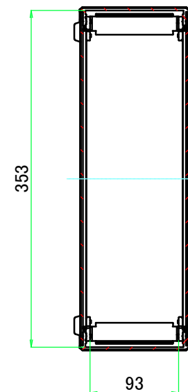
A-A ( 1 : 5.5 )
