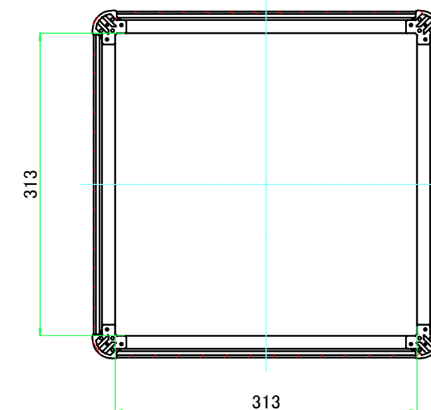
C-C ( 1 : 5.5 )
