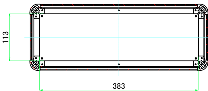
C-C ( 1 : 5.5 )
