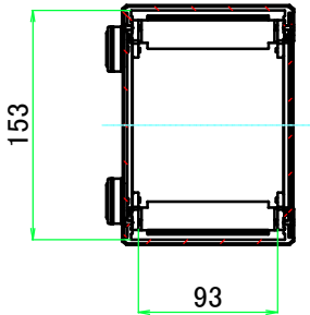
B-B ( 1 : 5.5 )
