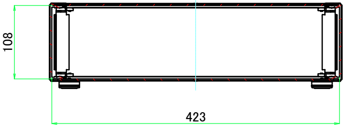
A-A ( 1 : 5.5 )
