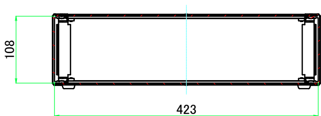
B-B ( 1 : 6 )
