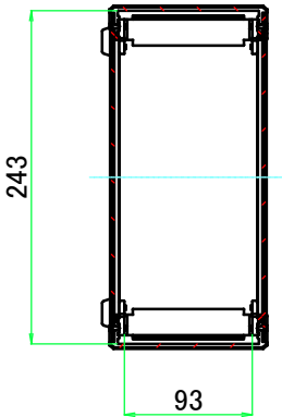
A-A ( 1 : 6 )
