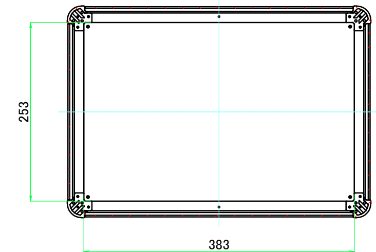
C-C ( 1 : 5.5 )
