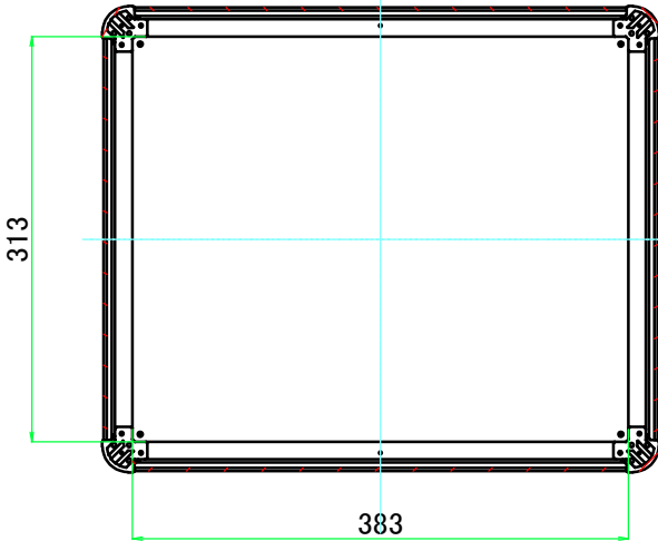
C-C ( 1 : 6.5 )
