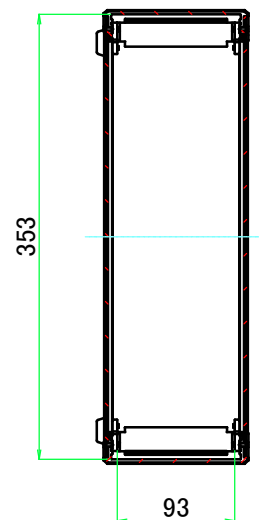
A-A ( 1 : 6 )
