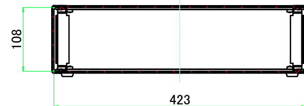
B-B ( 1 : 6.5 )
