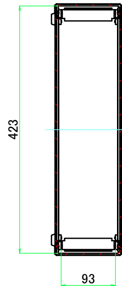
A-A ( 1 : 6.5 )
