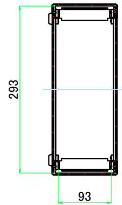
A-A ( 1 : 6.5 )
