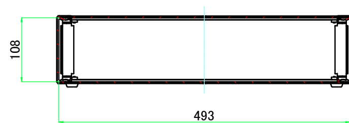
B-B ( 1 : 6.5 )
