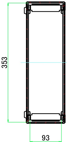
A-A ( 1 : 6.5 )
