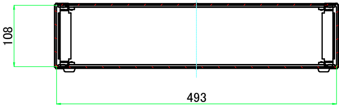
B-B ( 1 : 6.5 )
