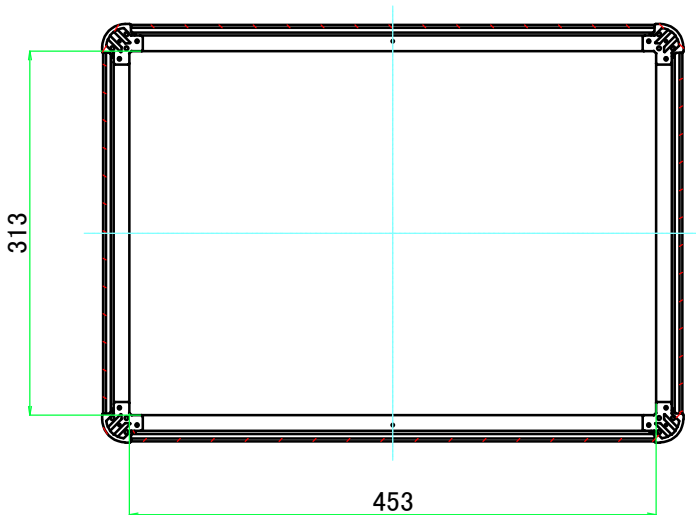
C-C ( 1 : 6.5 )
