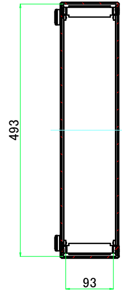
B-B ( 1 : 7.5 )
