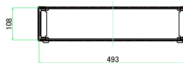
B-B ( 1 : 7.5 )
