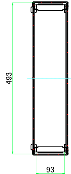
A-A ( 1 : 7.5 )
