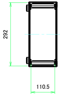
A-A (1 : 7.5)
