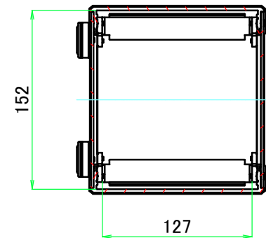
B-B ( 1 : 4.5 )
