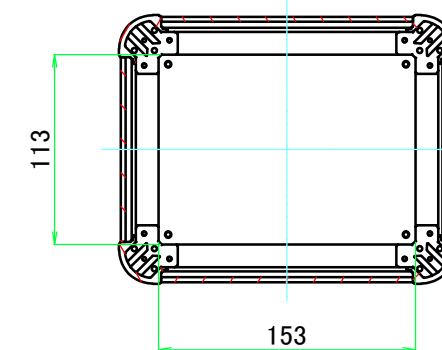
C-C ( 1 : 4.5 )
