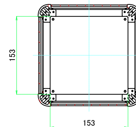
C-C ( 1 : 4.5 )
