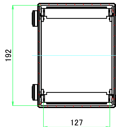
B-B ( 1 : 4.5 )
