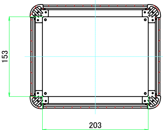
C-C ( 1 : 4.5 )
