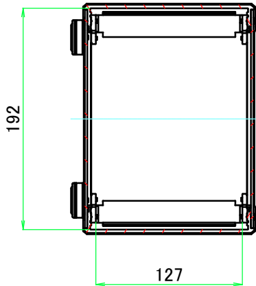
B-B ( 1 : 4.5 )
