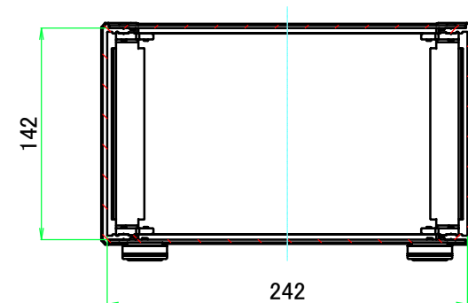
A-A ( 1 : 4.5 )
