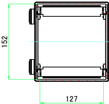
B-B ( 1 : 4.5 )
