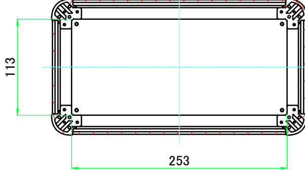
C-C ( 1 : 4.5 )
