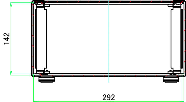
A-A ( 1 : 4.5 )
