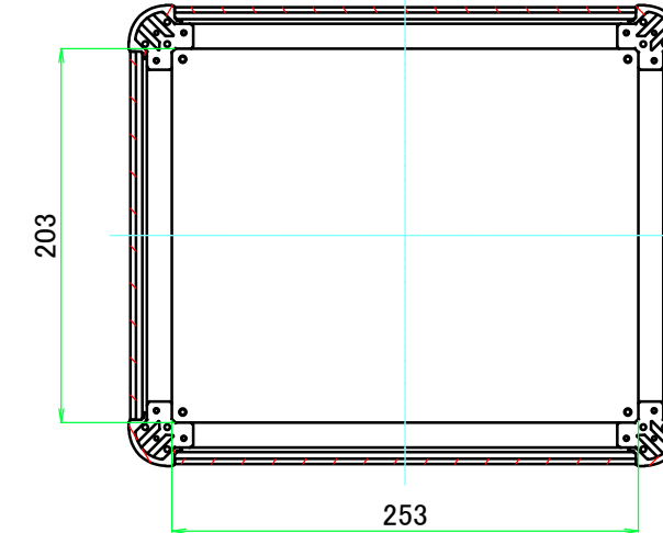
C-C ( 1 : 4.5 )
