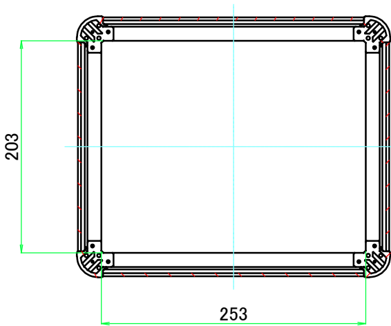
C-C ( 1 : 5 )
