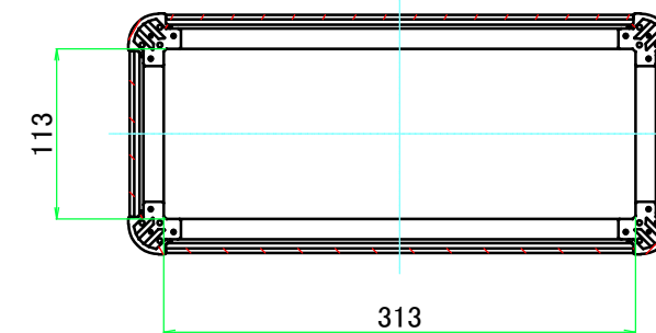
C-C ( 1 : 5.5 )
