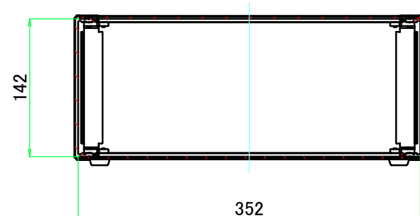
B-B ( 1 : 5.5 )
