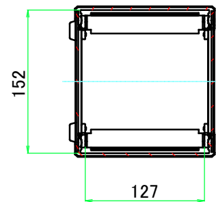
A-A ( 1 : 5.5 )
